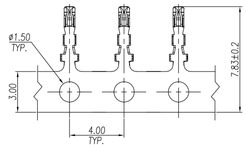
排样图 SC 0.25:1
