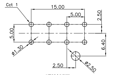
C型基板示意图
