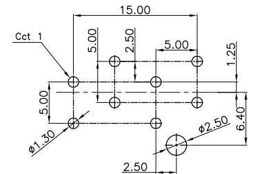
A型基板示意图
