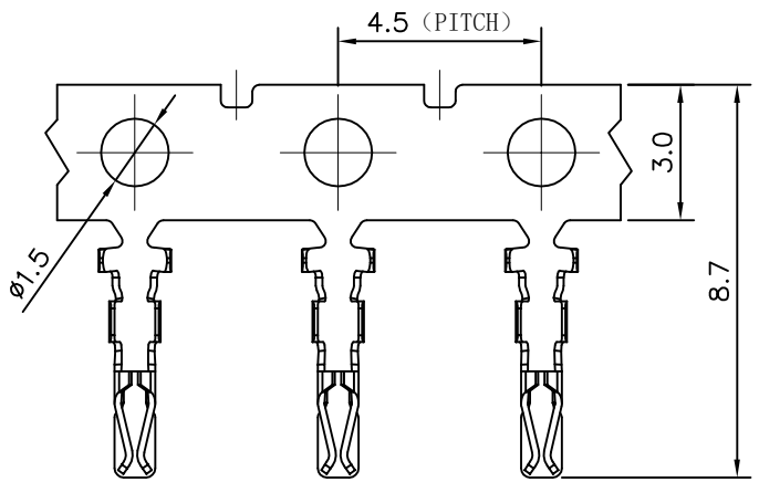
排样图 SCALE 0.5:1
