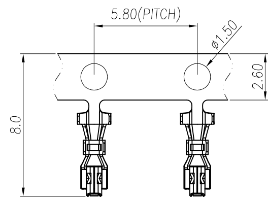
排样图 SCALE 0.5:1
